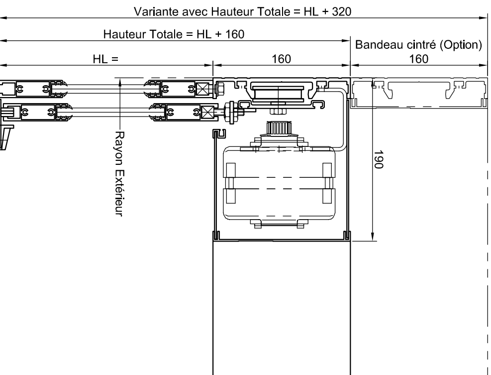
Détail Coupe Verticale AA Vantail coulissant mis dans le plan de coupe
