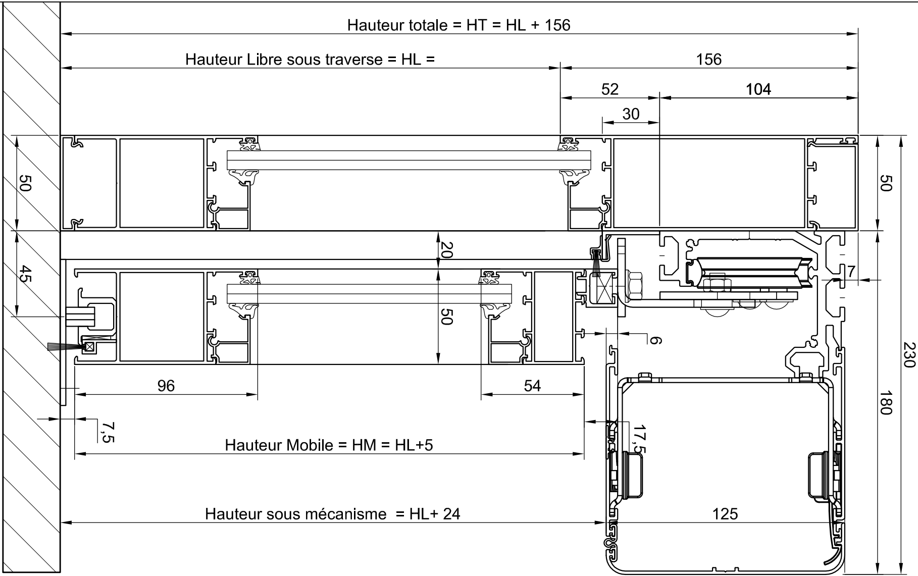
Coupe sur partie fixe
