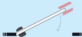
Simple vantail
